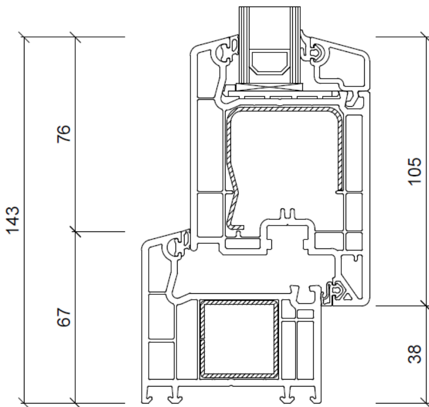
otevíravé dovnitř
