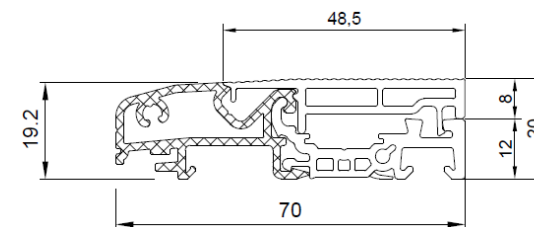
AL práh (104.427)
