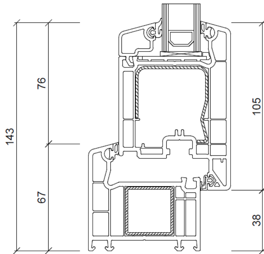
otevíravé ven
