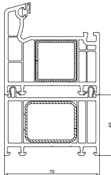
114.202 – Rozšíření 45mm
