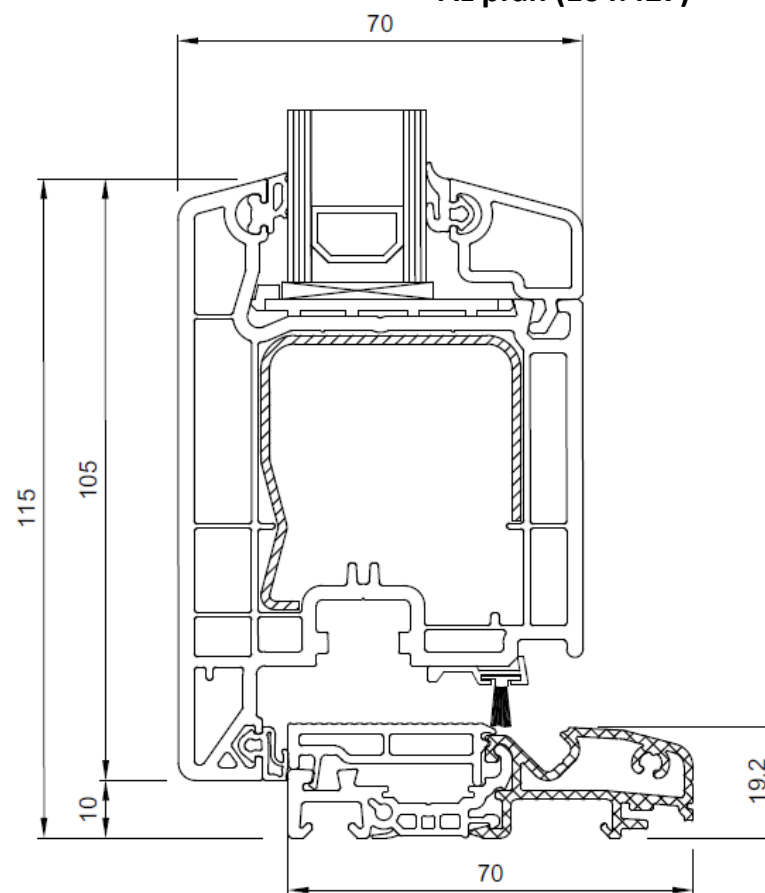
otevíravé ven
