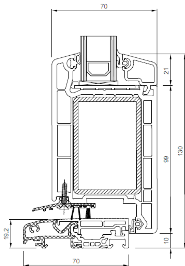
otevíravé dovnitř
