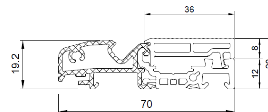
AL práh (104.427)
