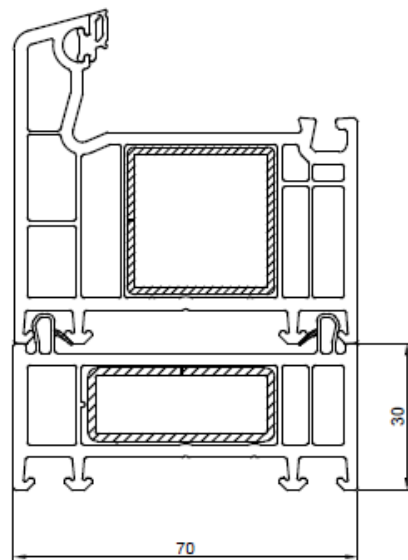
114.201 – Rozšíření 30mm
