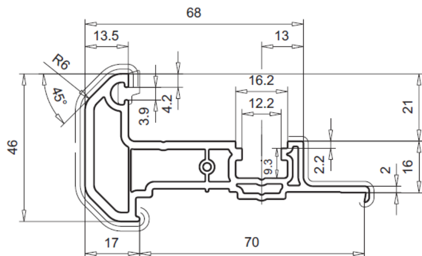
102.219
