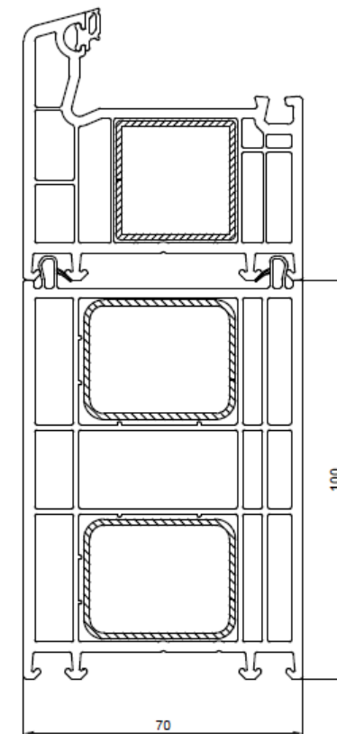
114.203 – Rozšíření 100mm
