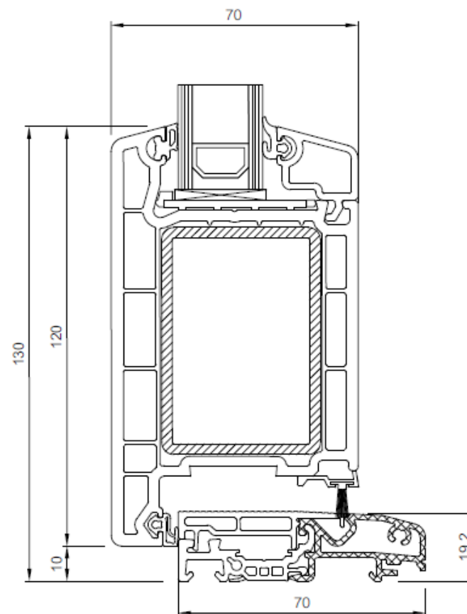
AL práh (104.427)
